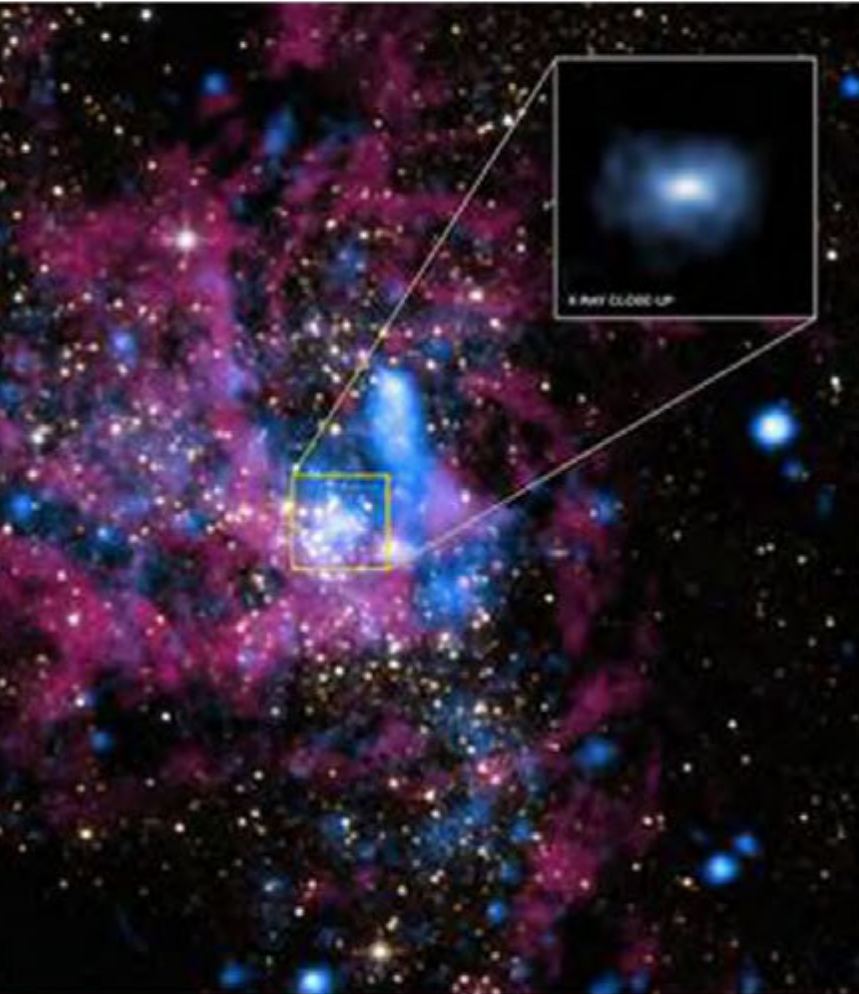
(Samanyolu galaksisinin merkezinde Yay A'nın bu görüntüsü, Chandra X-ray Gözlemevi tarafından alındı.) NASA / CXC / MIT / FK Baganoff ve ark.
